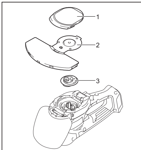
► 1. Sous-couvercle 2. Lames de cisaillement 3. Manivelle
