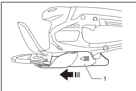
► 1. Collecteur d'herbes
