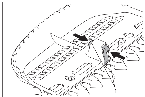
► 1. Leviers
