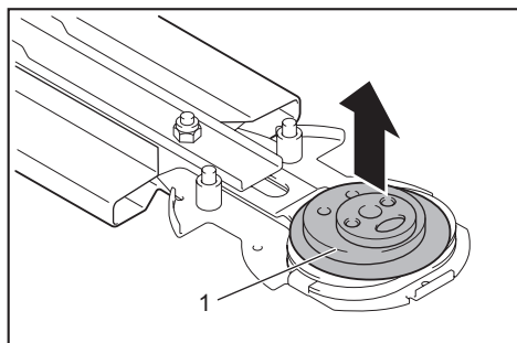
► 1. Manivelle
